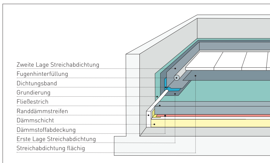
Streichabdichtung
